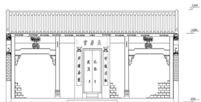
图3 淇澳岛天后宫立面图
