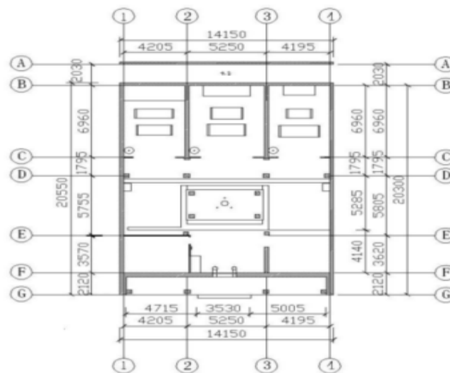
图4 淇澳岛天后宫建筑平面图
